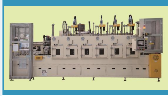
6조 자동 초음파+스프레이 세척기 (Loading Room, Unloading Room)
