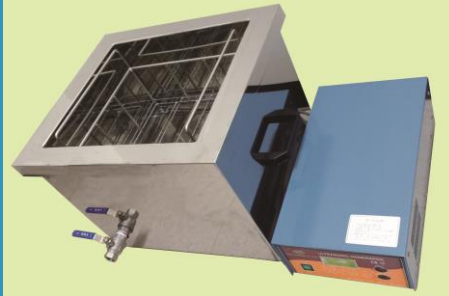
1조식 분리형 초음파 세척기 (발진부 분리형 TYPE)
